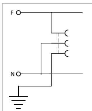
Esquema multifilar
